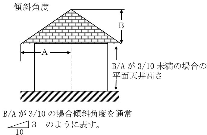
傾斜天井の角度、面積、平均高さの出し方
