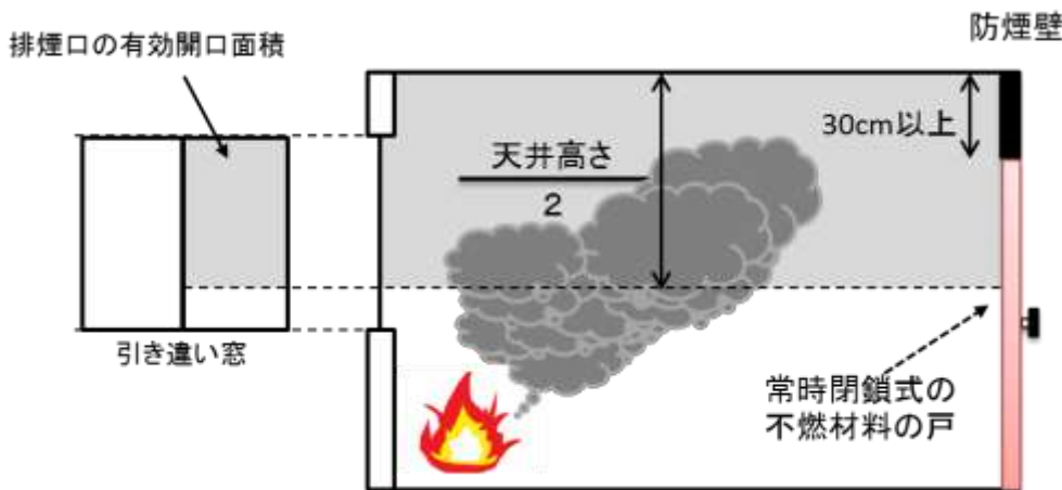
第 19-13 図 イの例（防煙壁に常時閉鎖式の不燃戸を設けた場合の有効開口面積）
