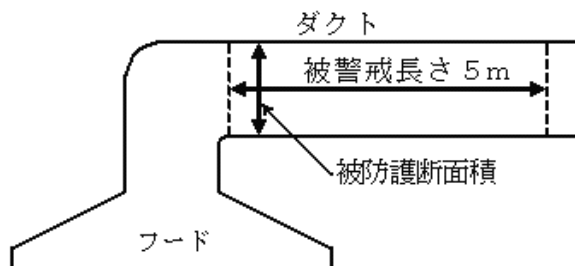
第 24-4 図 ダクトの被警戒長さ及び被防護断面面積
