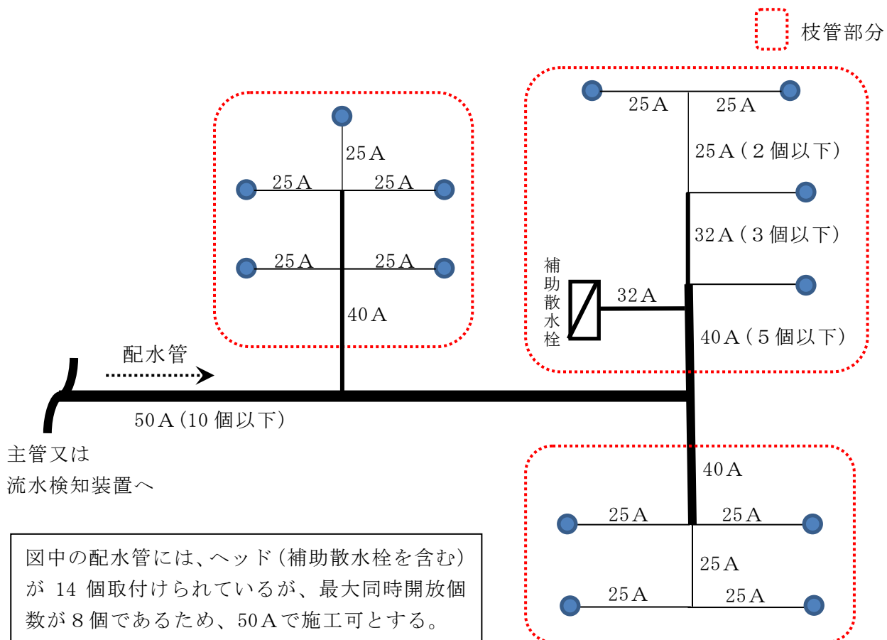
第 4-4 図 配置の設置例：標準型ヘッド(最大同時開放個数 8 個)の場合
