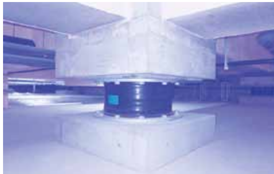
▲免振構造部分 建物の基礎部分にゴム層を入れ、振動が建物に伝わりにくい構造になっています。
